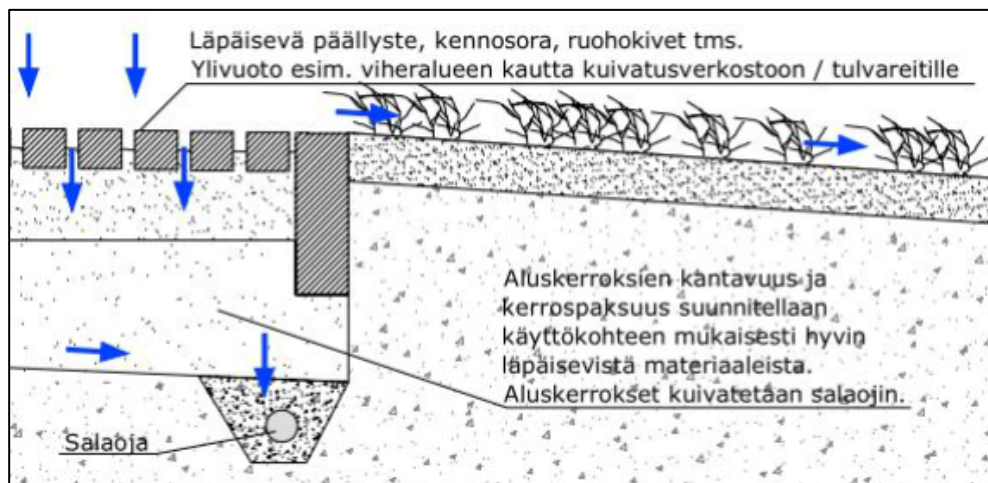
Kuva 16. Tyypikuva läpäisevästä pintarakenteesta pysäköintialueella
